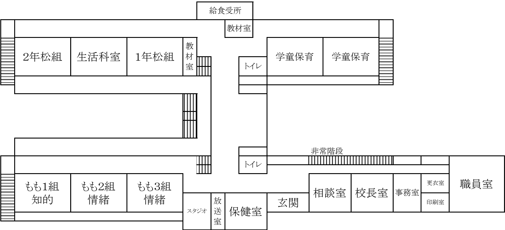
1 階 平 面 図
